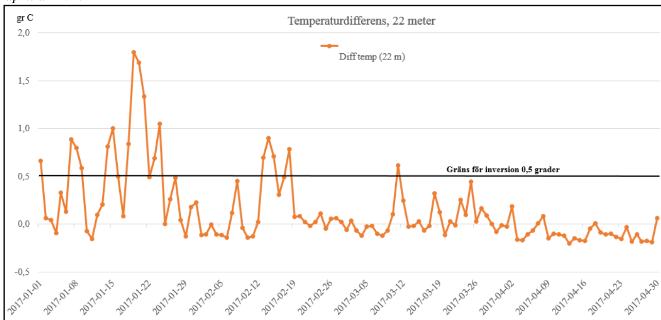
Figur 3: Dygnsmedelvärden av temperaturdifferens vid masten i Falun, 1:a januari till 30:e april år 2017
